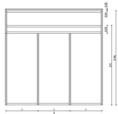
VISTA FRONTAL OPTICO PLACA. 0.95 M X 2.375 M OPTICO CENEFA. 2.93 M X 0.241 M
