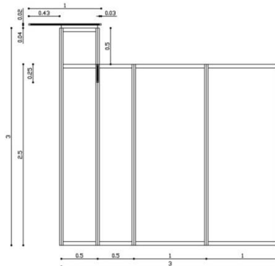
VISTA LATERAL OPTICO PLACA. 0.95 M X 2.375 M OPTICO CENEFA. 2.93 M X 0.241 M
